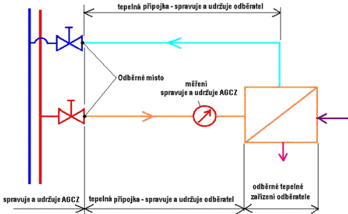
Schematické znázornění připojení odběrného místa zákazníka Alpiq Generation (CZ) s.r.o.
